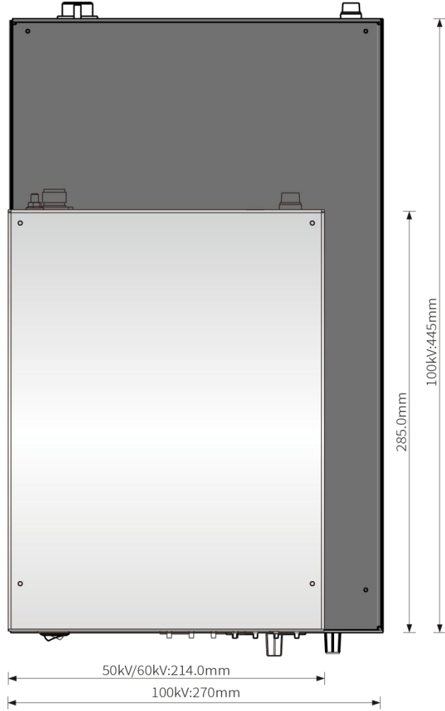
俯视图
