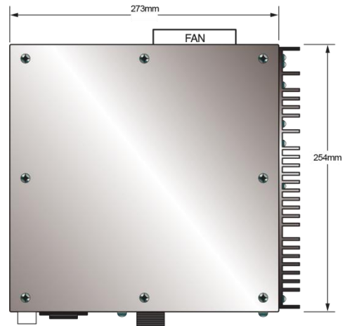
主视图
