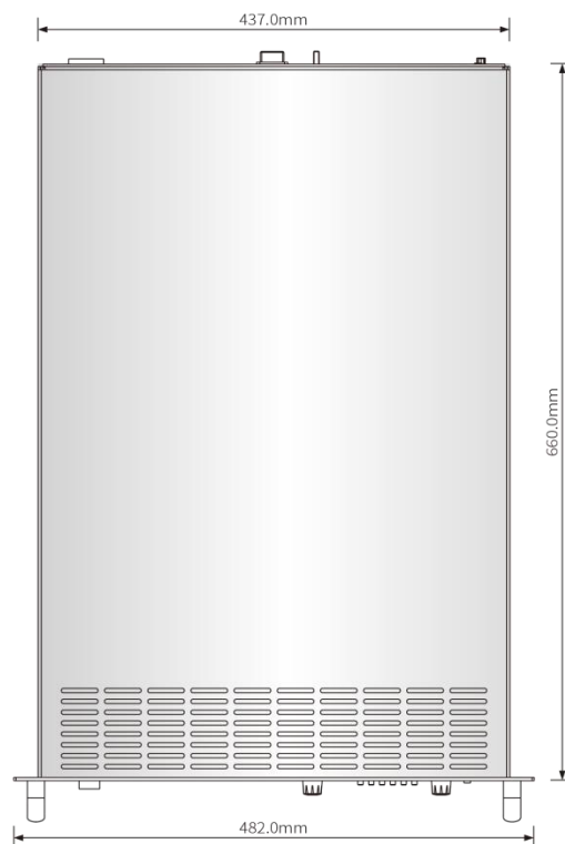
俯视图
