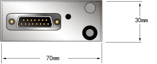
主视图
