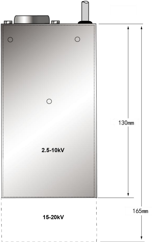
俯视图
