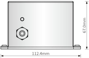
后视图
