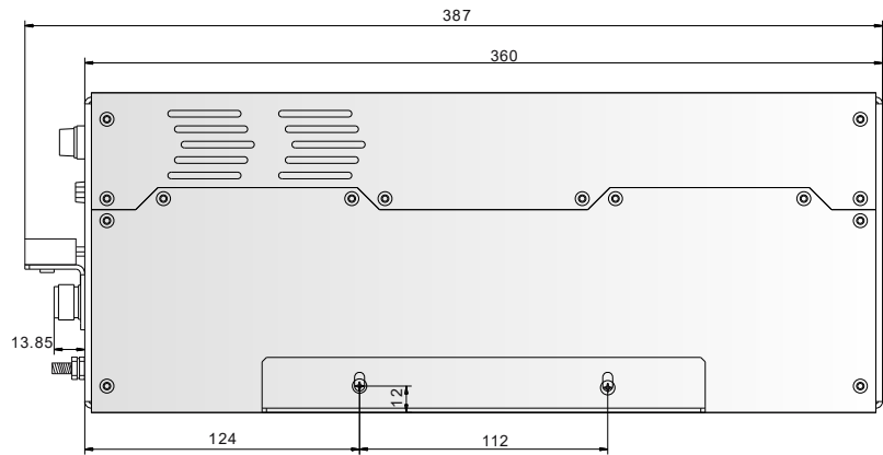
侧视图
