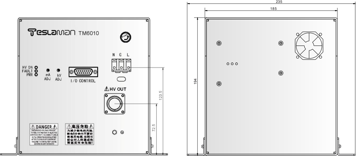
主视图
