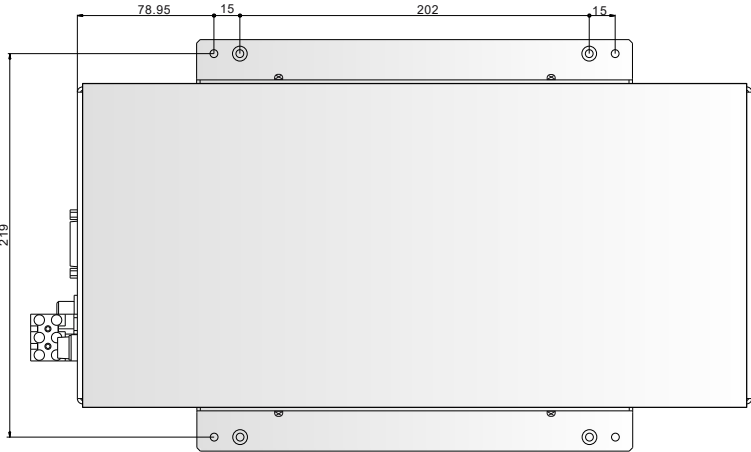
俯视图
