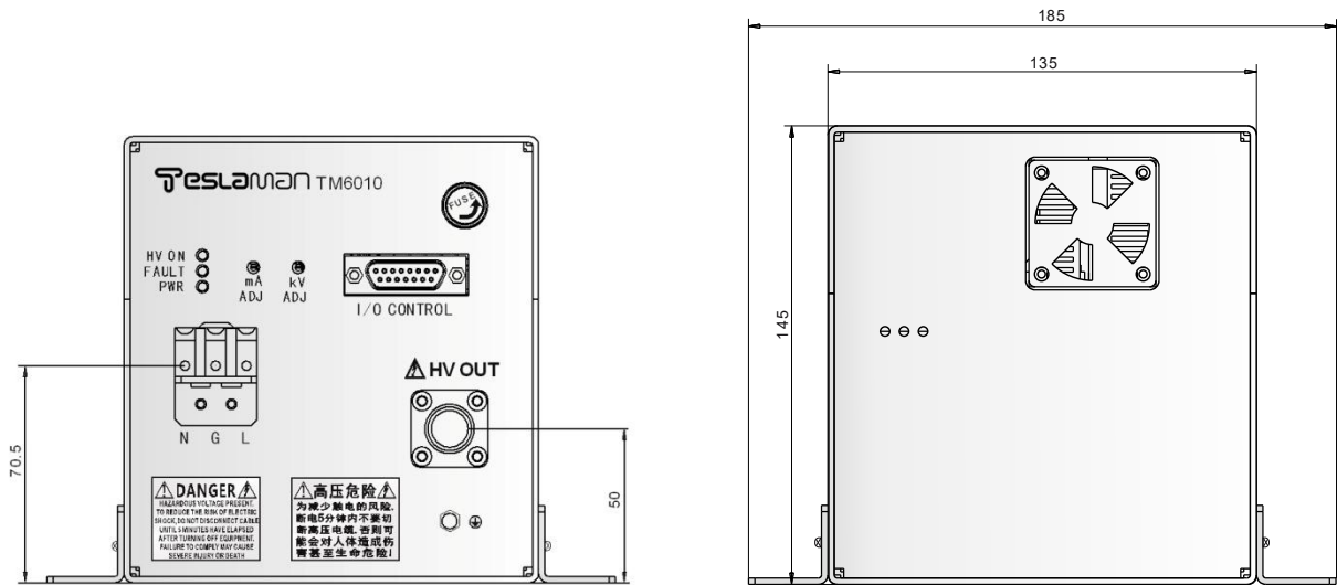
主视图
