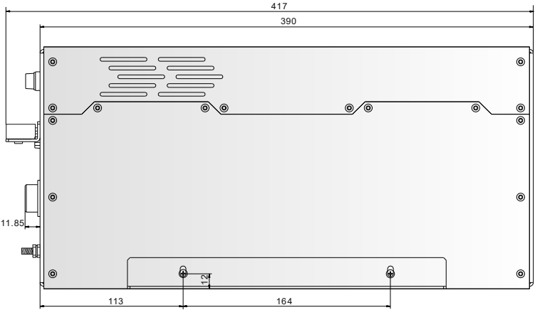
侧视图
