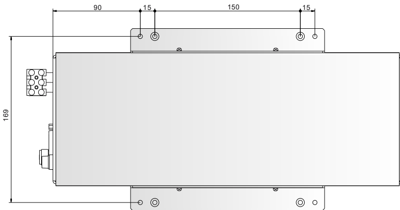
俯视图
