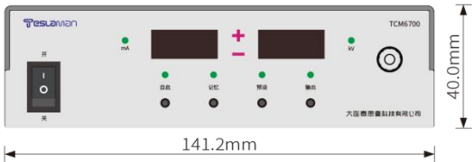
主视图
