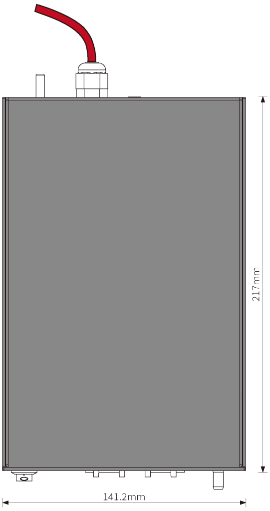
俯视图
