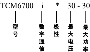
TCM6700 系列高压电源型号选择表（可定制）：
