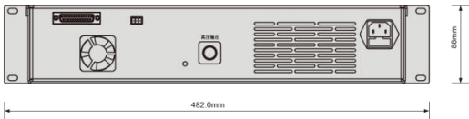
后视图
