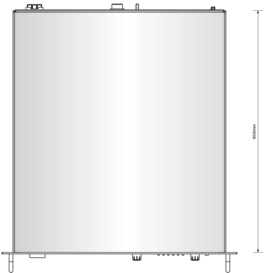
俯视图
