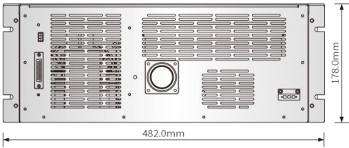
后视图
