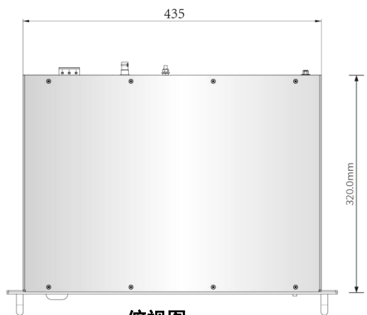
俯视图
