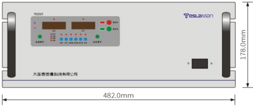
主视图
