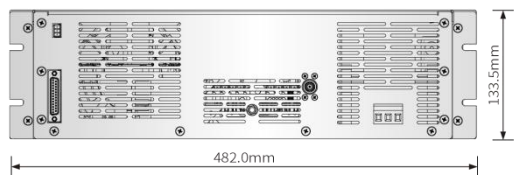
后视图
