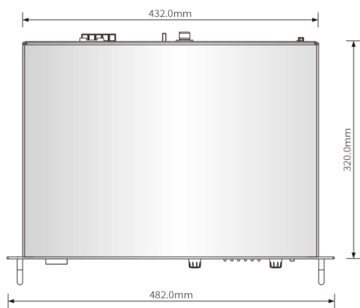
俯视图
