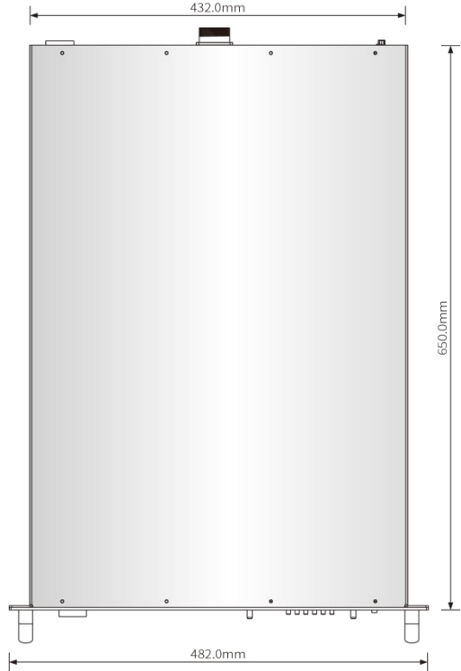
俯视图
